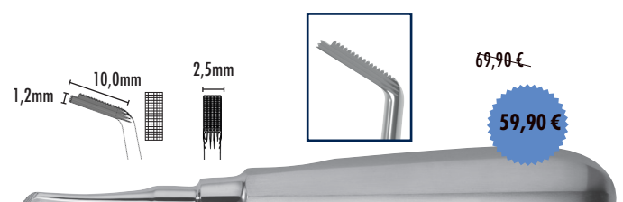
OLS-6101 Ligaturen-Zange gerade lingual MATHIEU-Zange gerade lingual - Das feine und gerade Arbeitsende der Zange ist optimal für die Bogen- und Ligaturen-Platzierung
